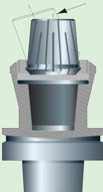
Sistema per sostituzione pinza Spring collect changing system Entfernen der Spannzangen
